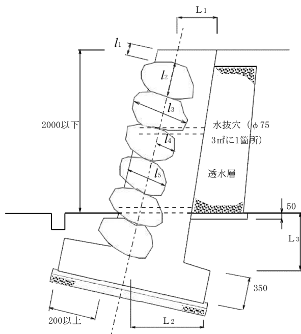
ア 玉石積 図 3-32
