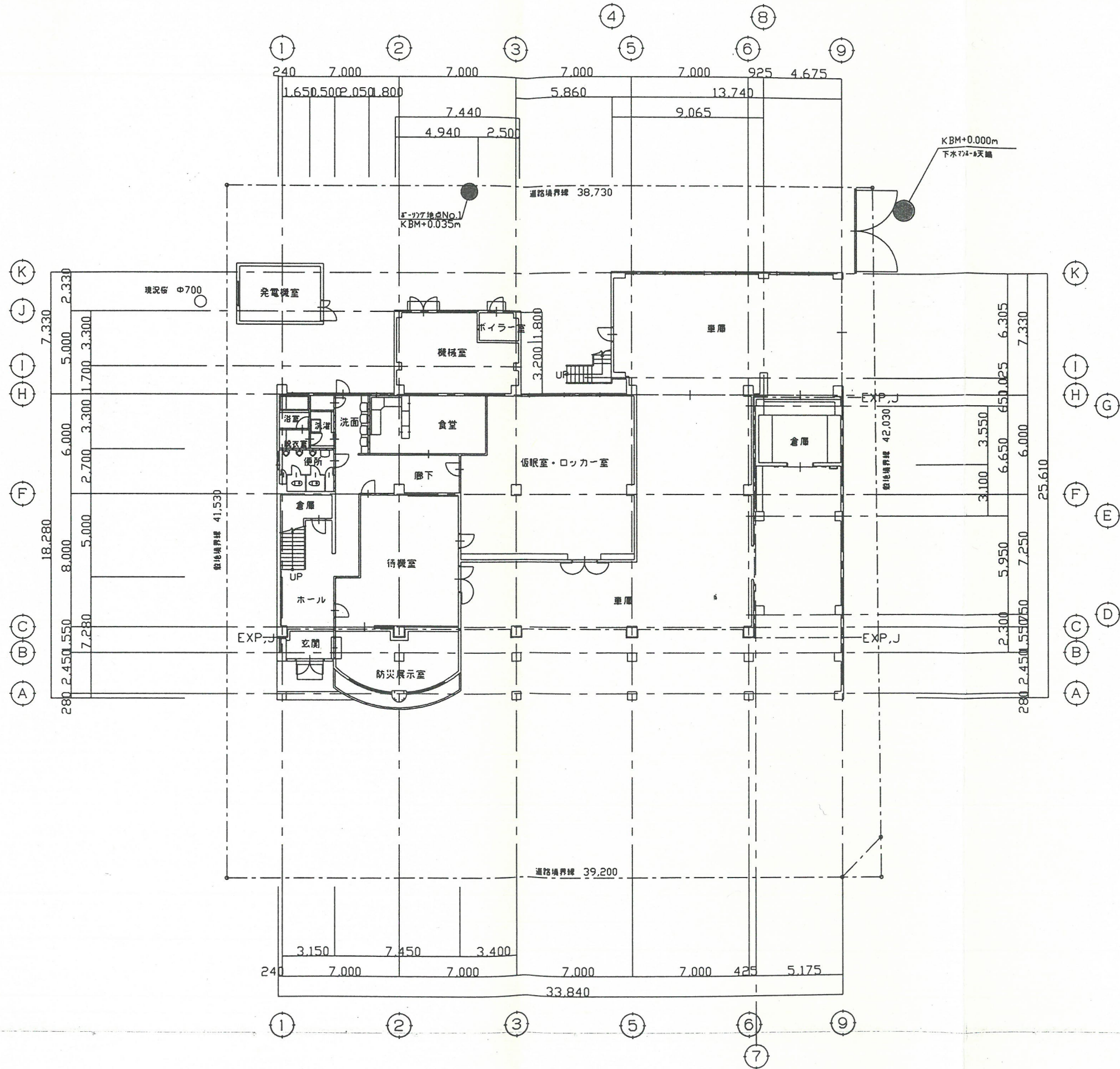
調査位置平面図 (縮尺 1:200)
