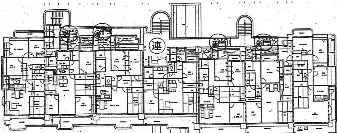
2~8階平面図
